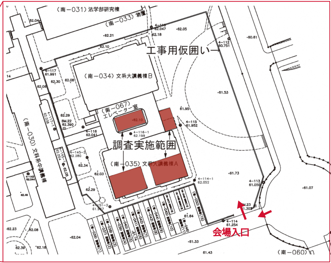
詳細図
